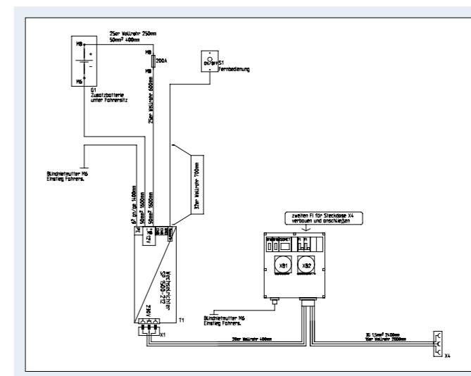
Eksempel på et kredsløbsdiagram
